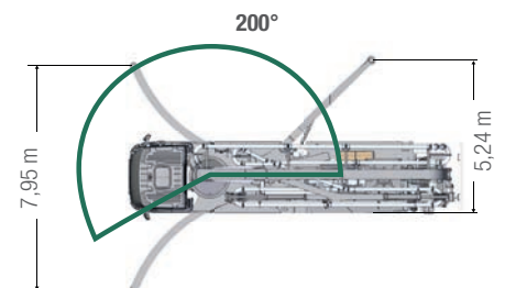
Teilabstützung (EASy 200)
